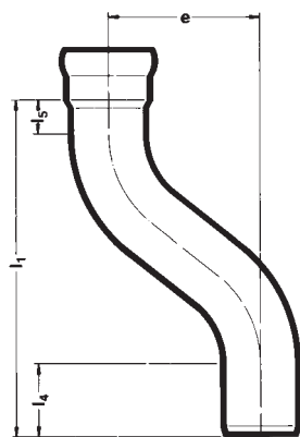
Tevi speciale e = 200 mm
