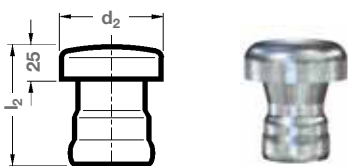
Sicherheitsdunsthüte mit Muffe für muffenlose Rohrenden
