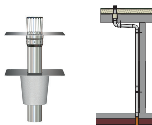
LORO-X Attikaentwässerung RAINSTAR® Distant Hochleistung mit Druckströmung, DN 100 Haupt- und Notentwässerung
