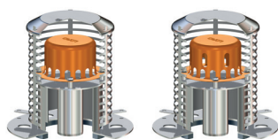
LORO-X Attikaentwässerung Haupt-Not-Kombi VARIOFIT Retentionseinheiten Freispeigelströmung und Druckströmung
