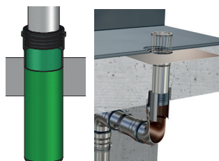
LORO-X Sanierungsdichtelemente für bestehende Abläufe oder Rohrleitungen
