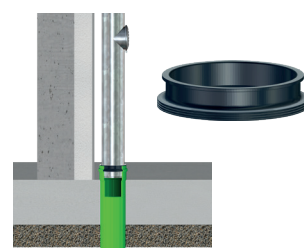
LORO-X Übergangsdichtelemente für Grundleitungen, aus Kunststoff
