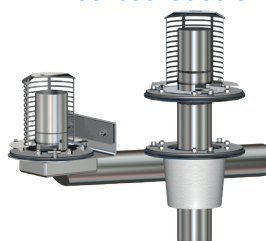
LORO-X Retentionsdrehchieber für Attikaabläufe und DRAINLET® Flachdachabläufe
