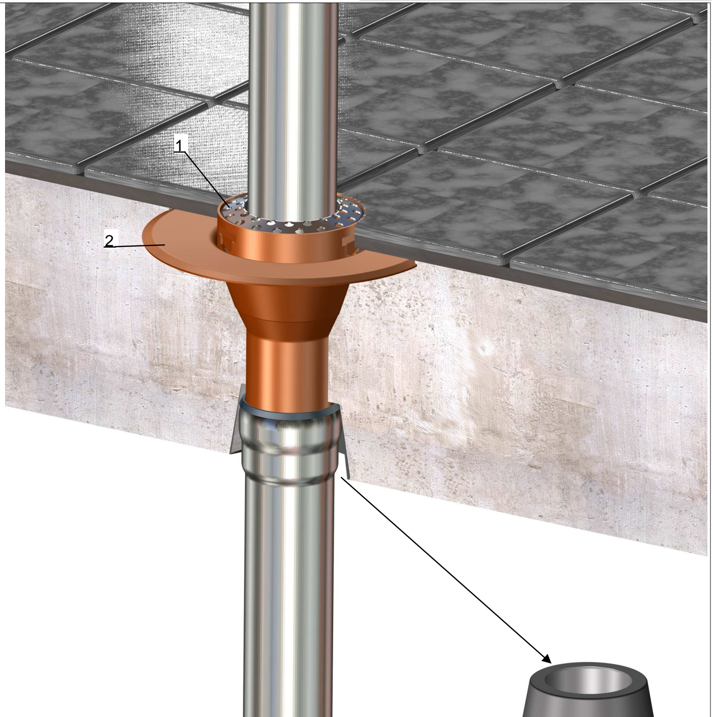
Balkondirektabläufe mit Stützrand Serie G für Balkone mit Fliesenbelag
