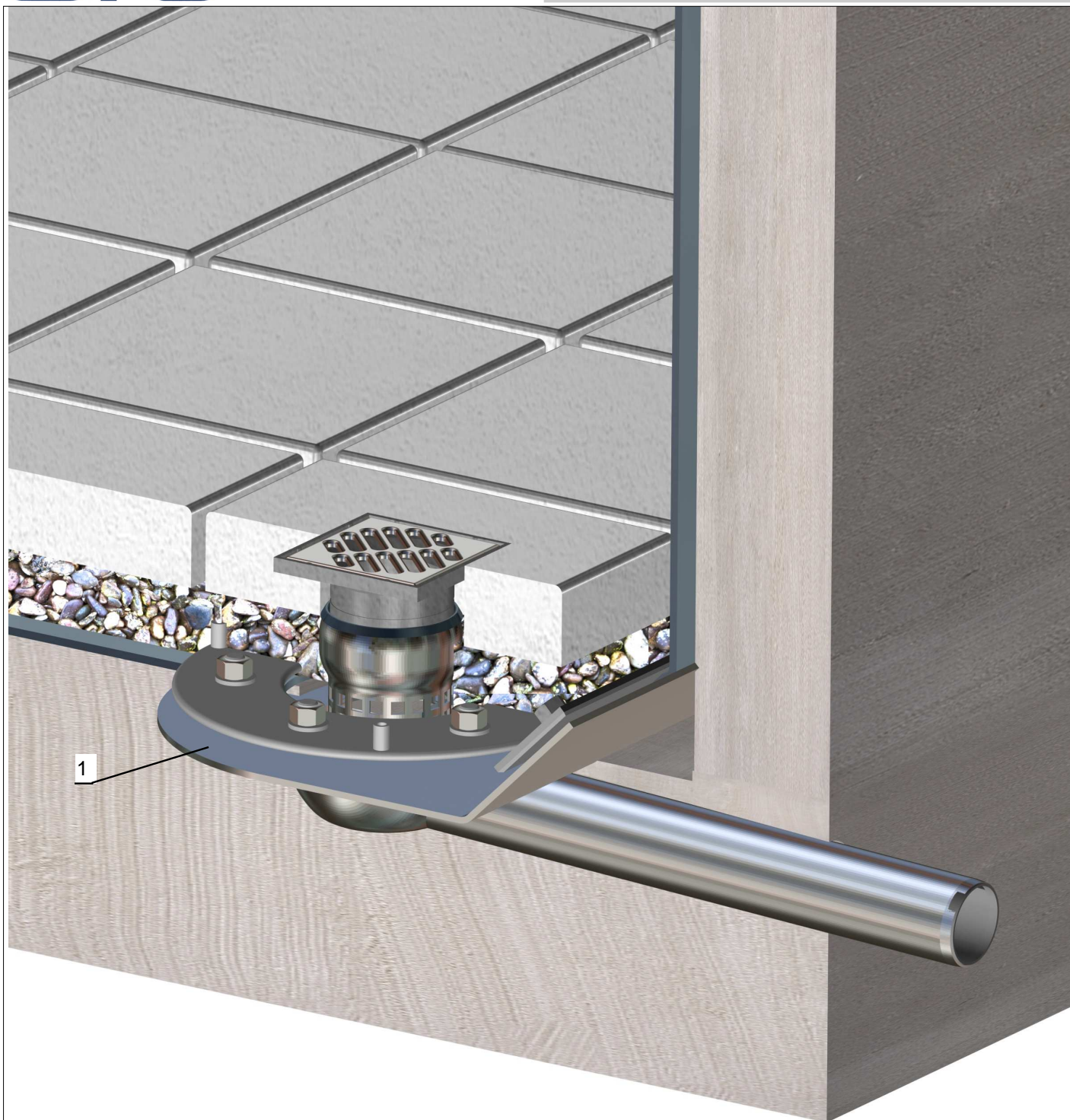
1 - LORO Attika-Balkonablauf mit Klemmflansch für Balkone mit Bitumen-Abdichtungsbahnen, Art.Nr. 01570.050X
