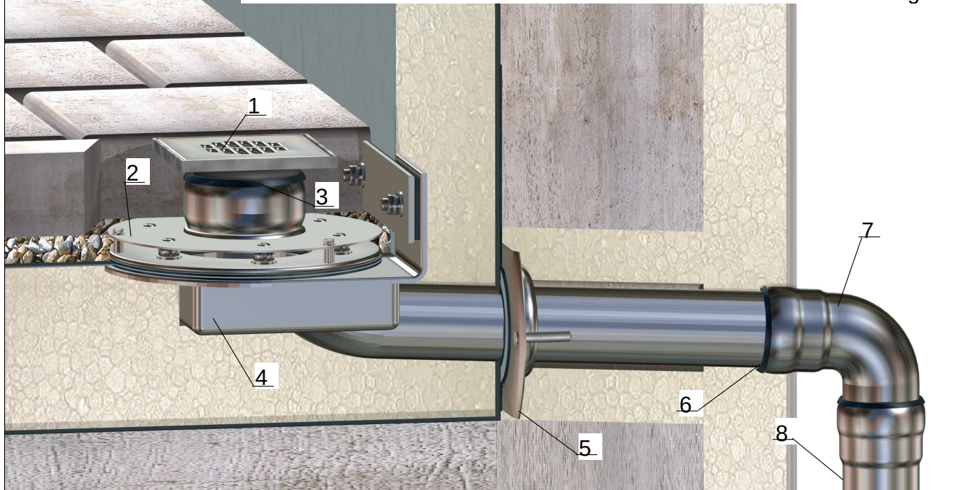
Bild10. Attikaablauf RAINSTAR mit Balkonablauf-Siebeeinheit und Sammelkasten
