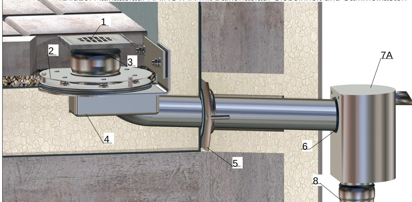
Bild10. Attikaablauf RAINSTAR mit Balkonablauf-Siebeeinheit und Sammelkasten
