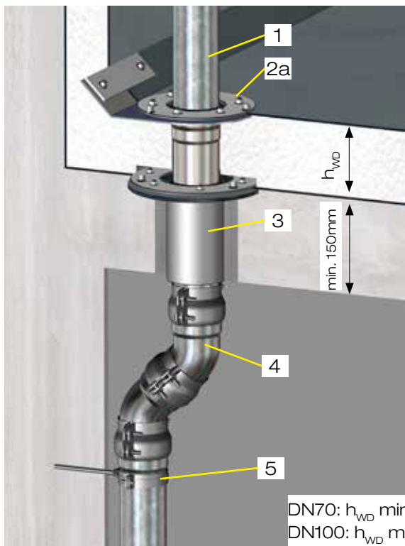
Bild 1. Rohrdurchführung senkrecht für Bitumenbahnen
