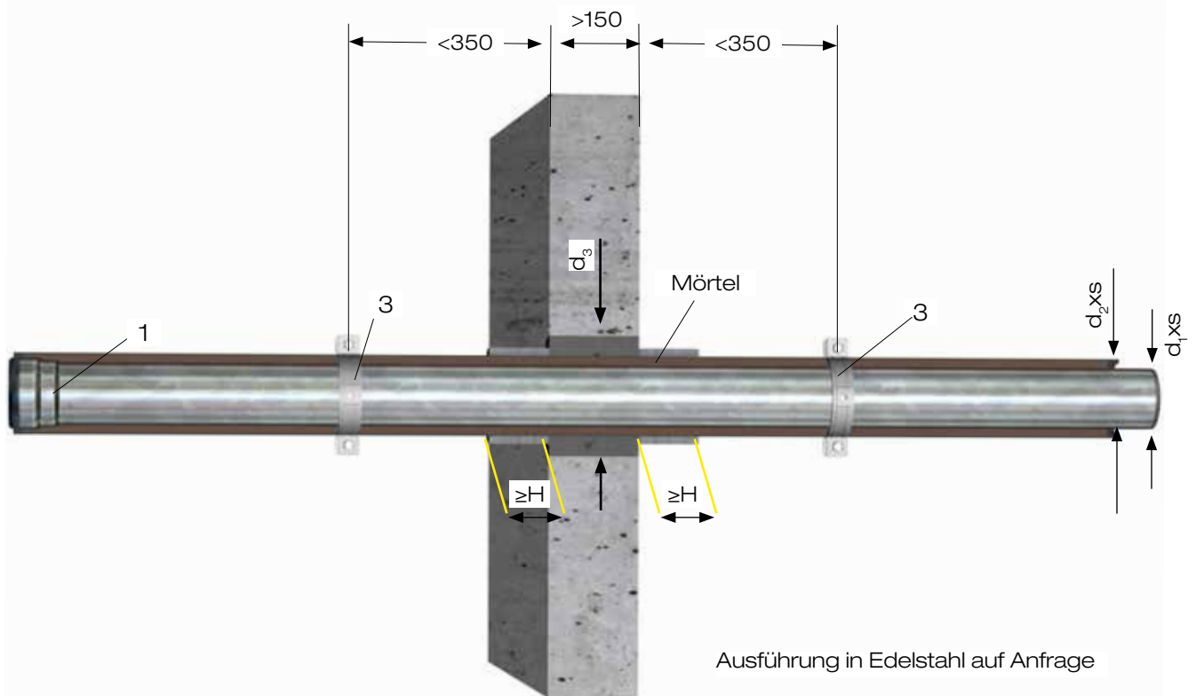
LORO-X Verbundrohr- Rohrdurchführung im Wandbereich
