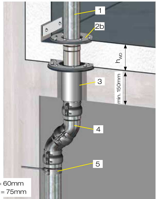
Bild 2. Rohrdurchführung senkrecht für Folienbahnen
