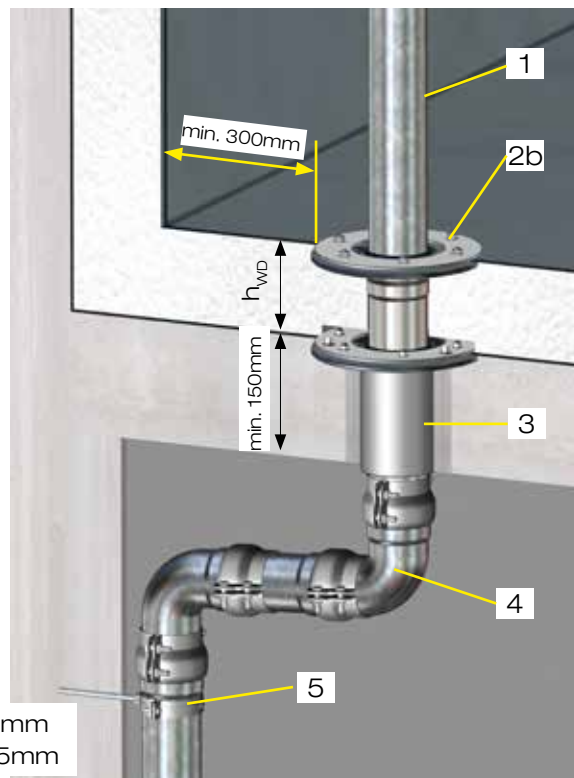
Bild 4. Rohrdurchführung senkrecht mit DRAINLET-Rohrdurchführung
