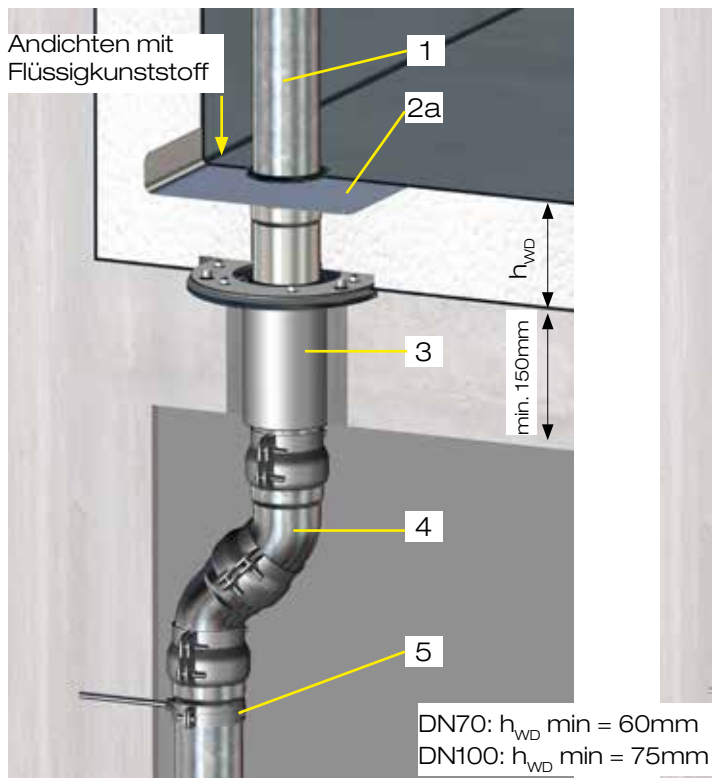
Bild 3. Rohrdurchführung senkrecht mit abkantbarem VARIO Kant Speier
