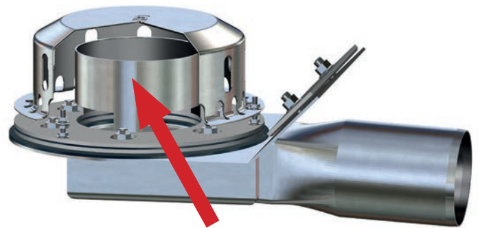
Drosselwehr
