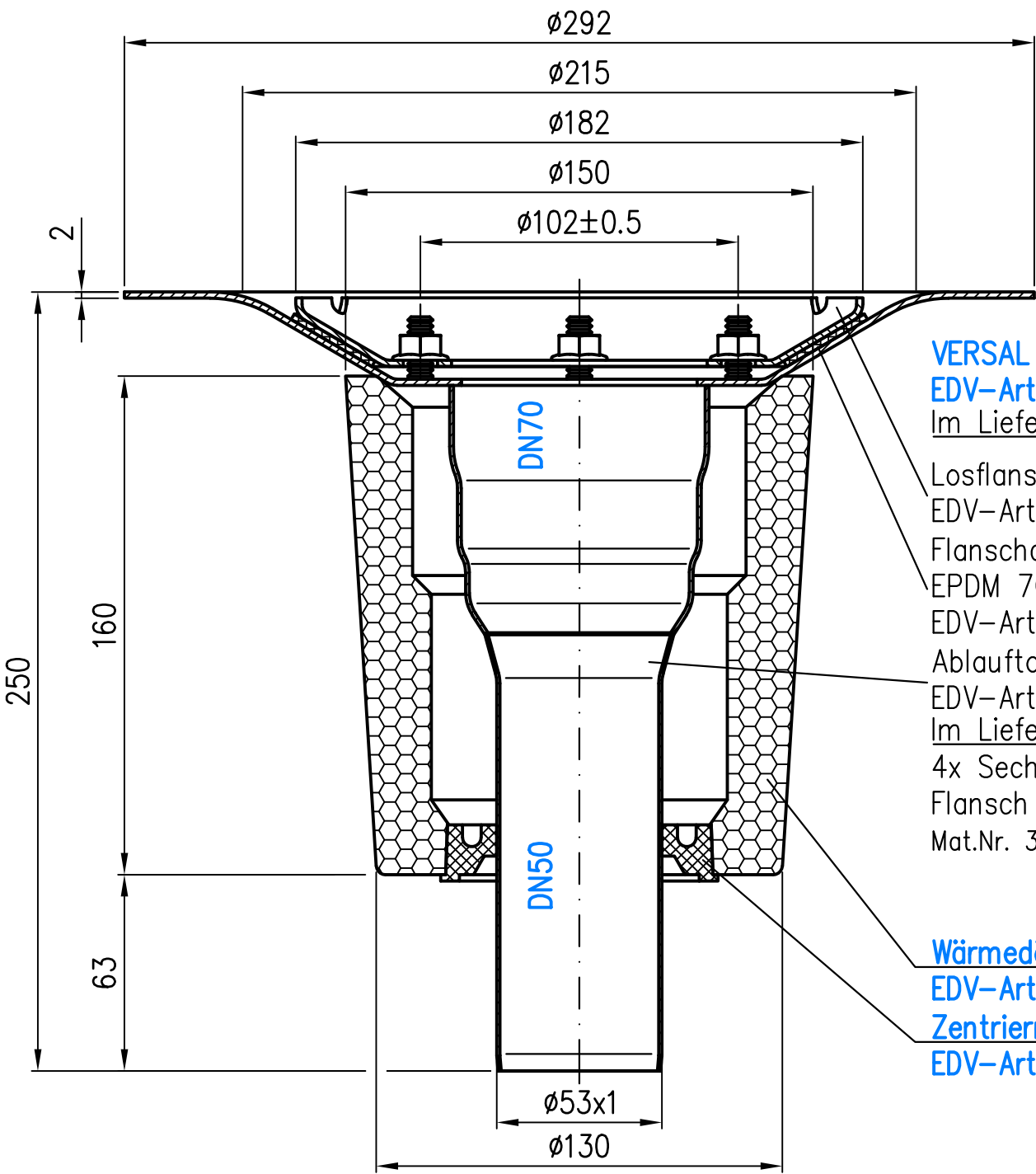
SCHNITT A-A
