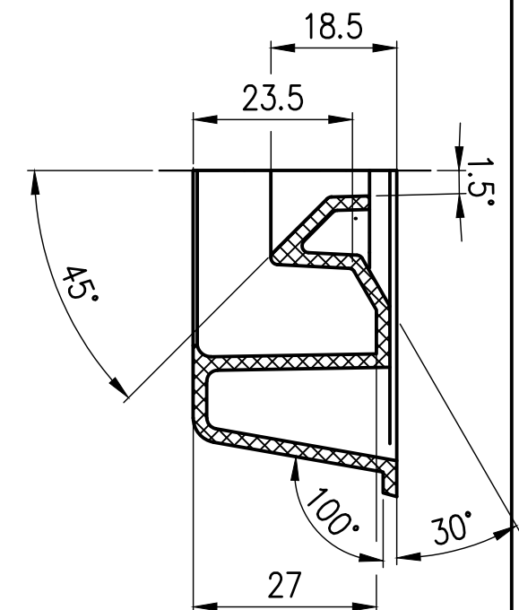
Schnitt: D-D Maßstab: 1:1
