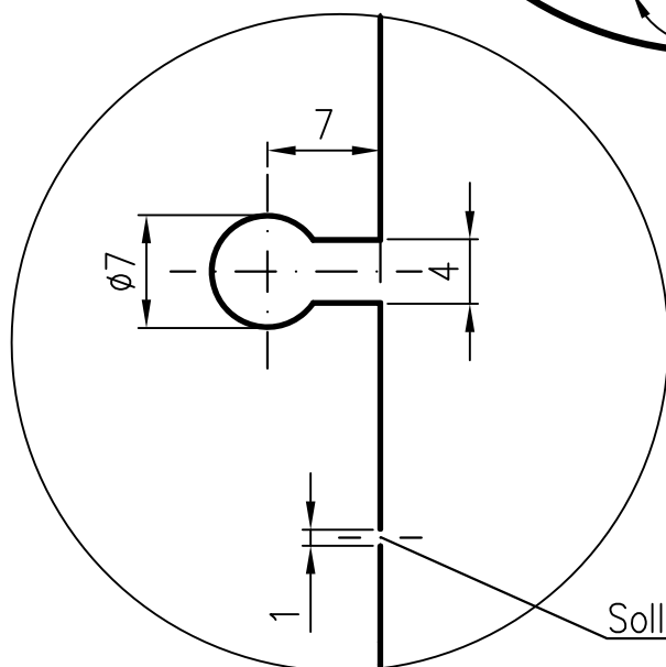
DETAIL B 2:1
