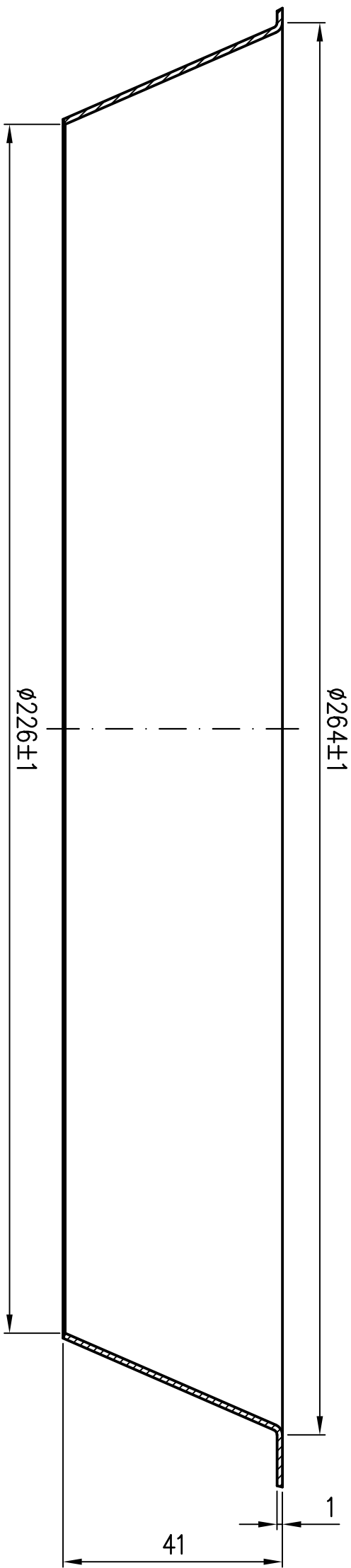
DETAIL Z Maßstab 1:1
