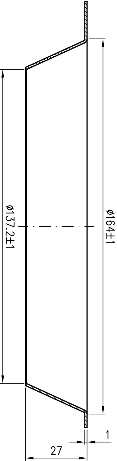
DETAIL Z Maßstab 1:1
