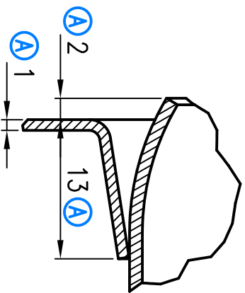
DETAIL Z Maßstab: 2:1
