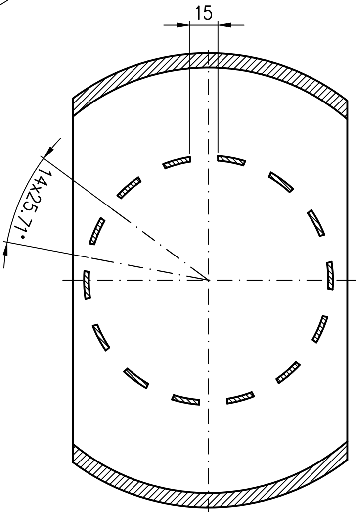
SCHNITT B-B
